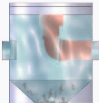
FIAP Vortex: Grobschmutzabscheider FIAP Vortex: coarse dirt separator
