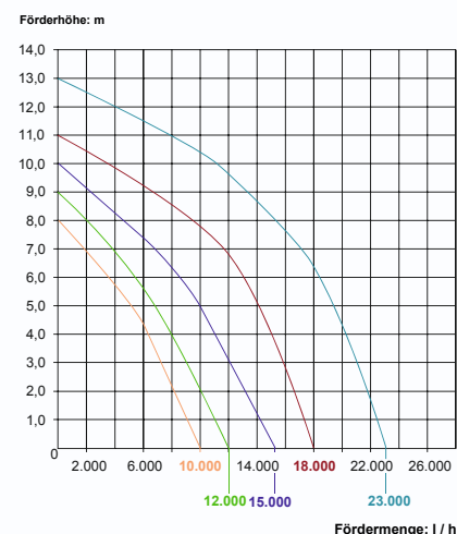
Pumpenkennlinien FIAP Aqua Active Magic
