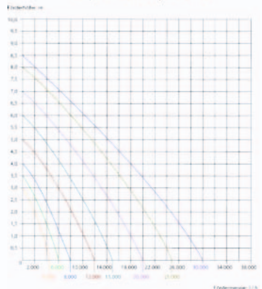
Pumpenkennlinie FIAP Aqua Active Profi
