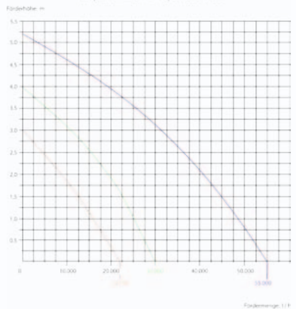
Pumpenkennlinie FIAP Aqua Active Power
